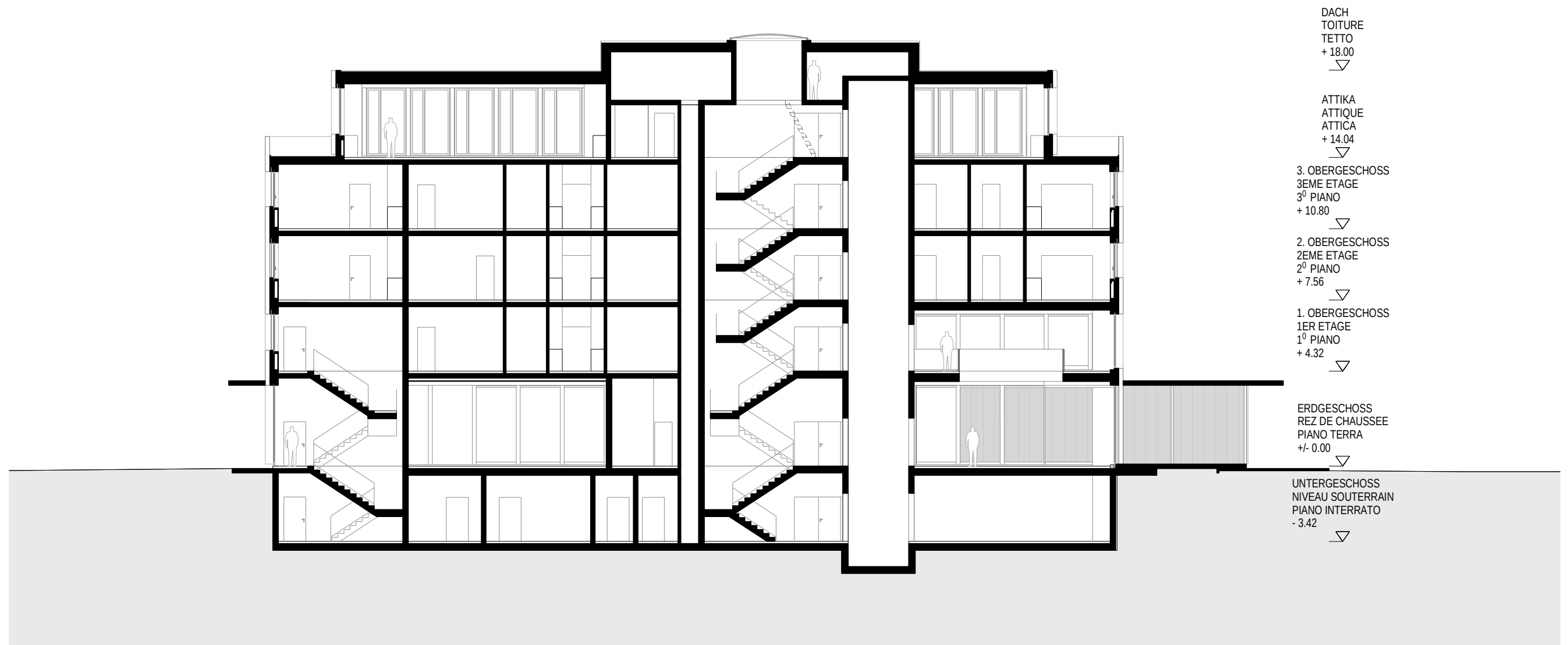
SCHNITT A-A COUPE A-A SEZIONE A-A
