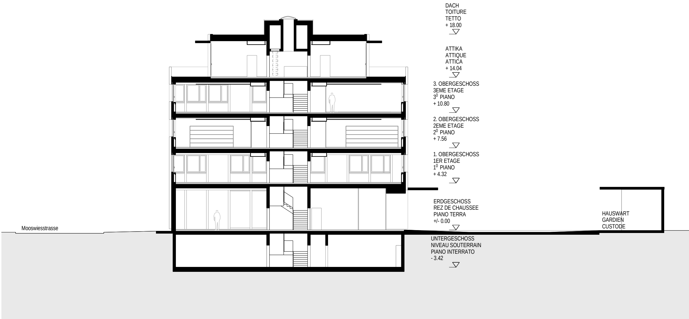
SCHNITT B-B COUPE B-B SEZIONE B-B
