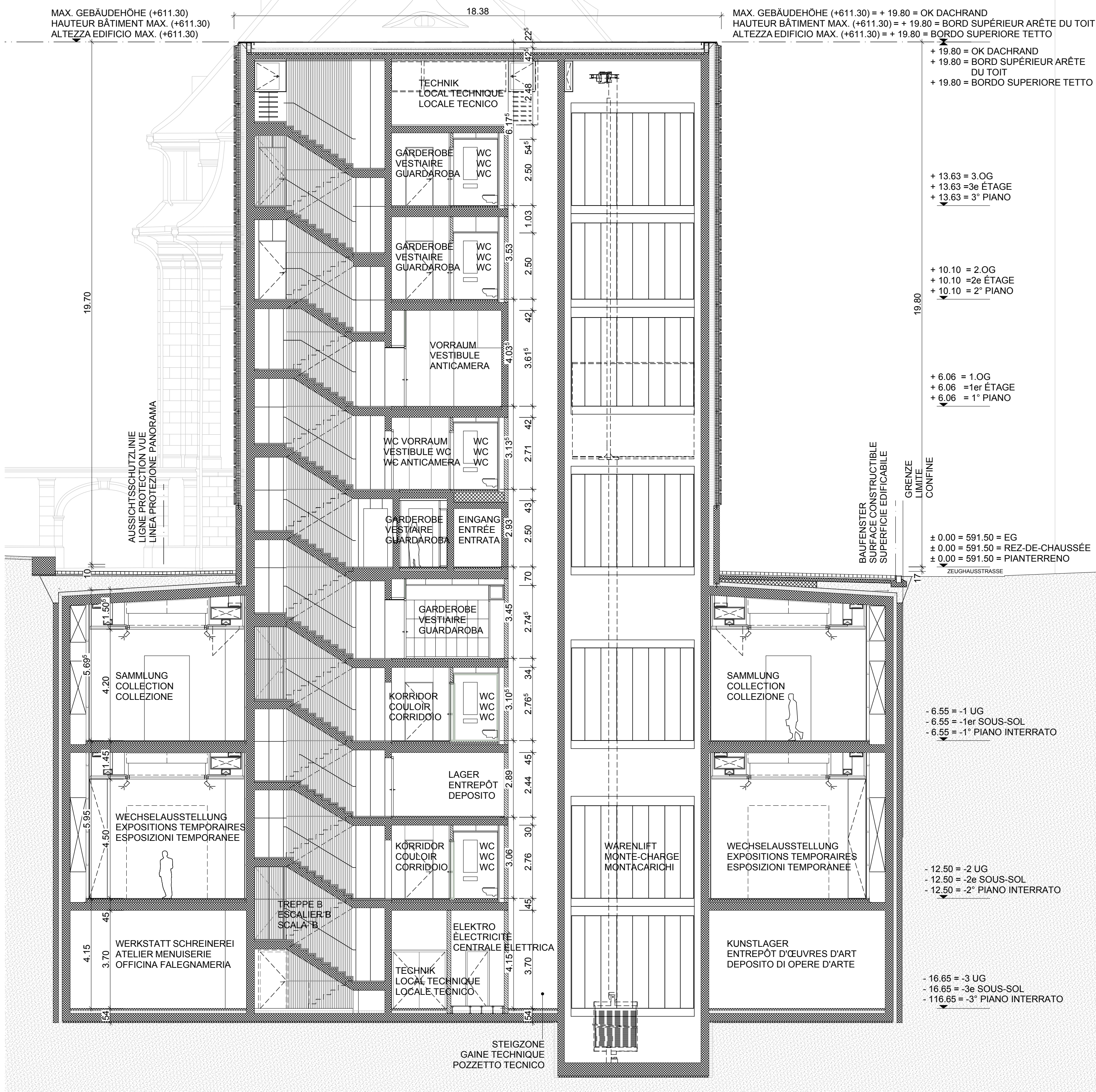
Schnitt L2 Taille L2 Sezione L2
