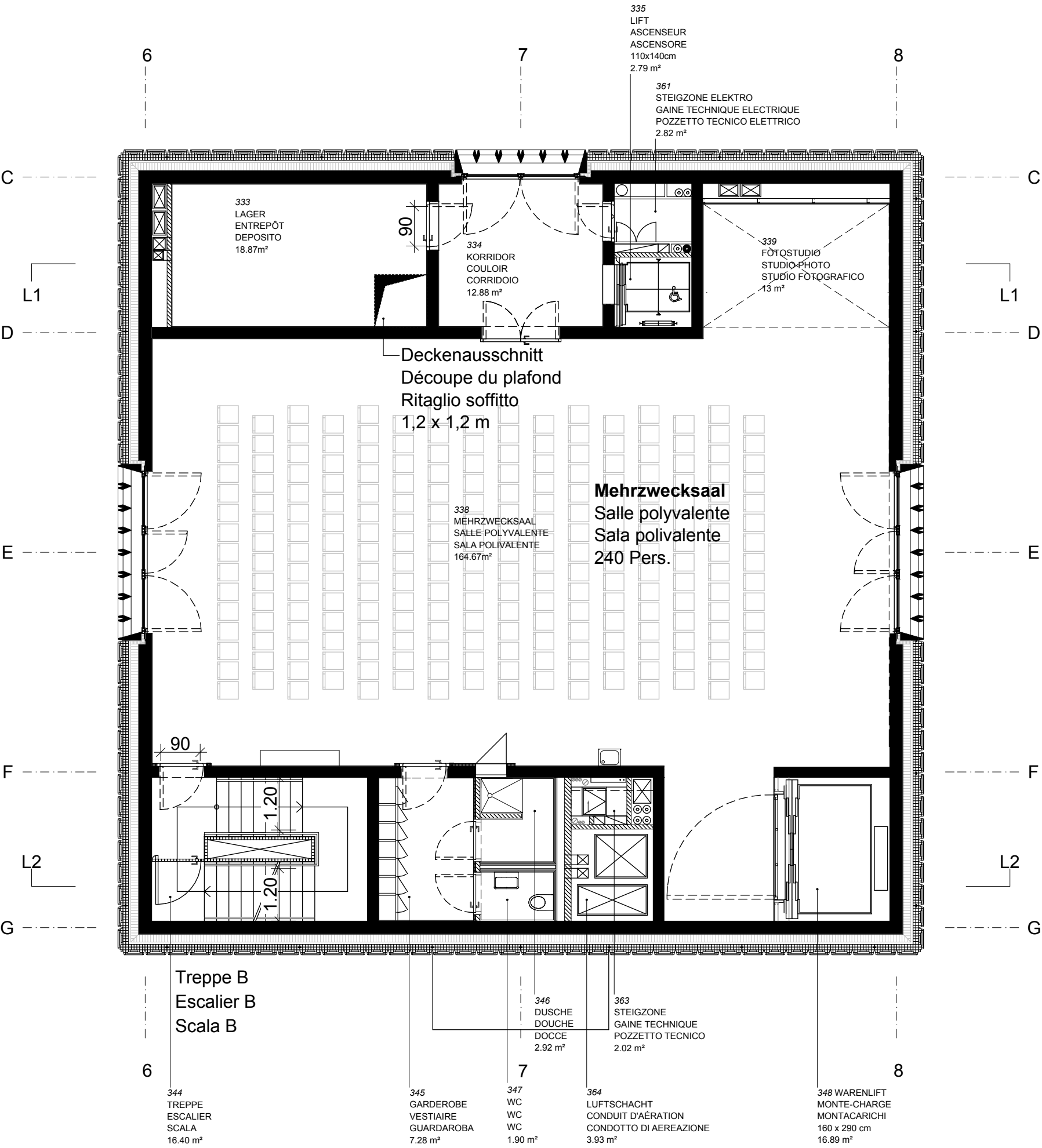
3. Obergeschoss 3e étage 3° piano
