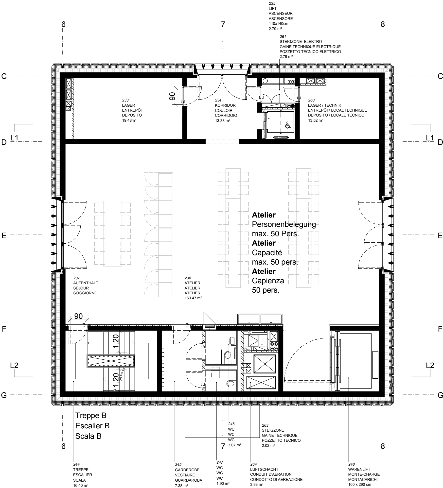
2. Obergeschoss 2e étage 2° piano
