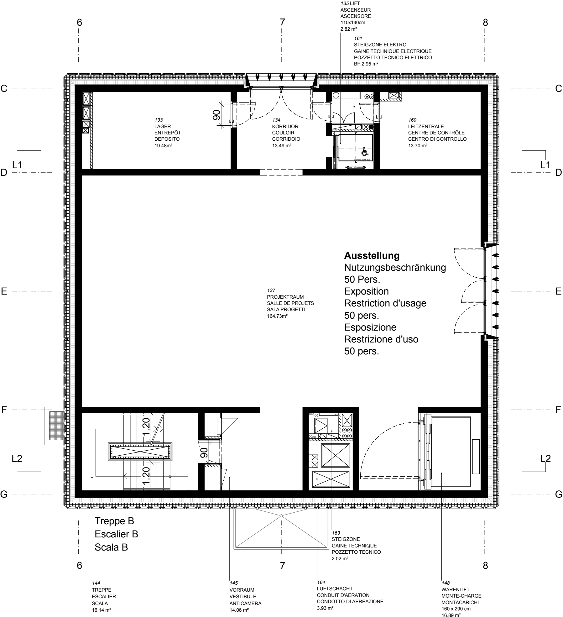
1. Obergeschoss 1er étage 1° piano
