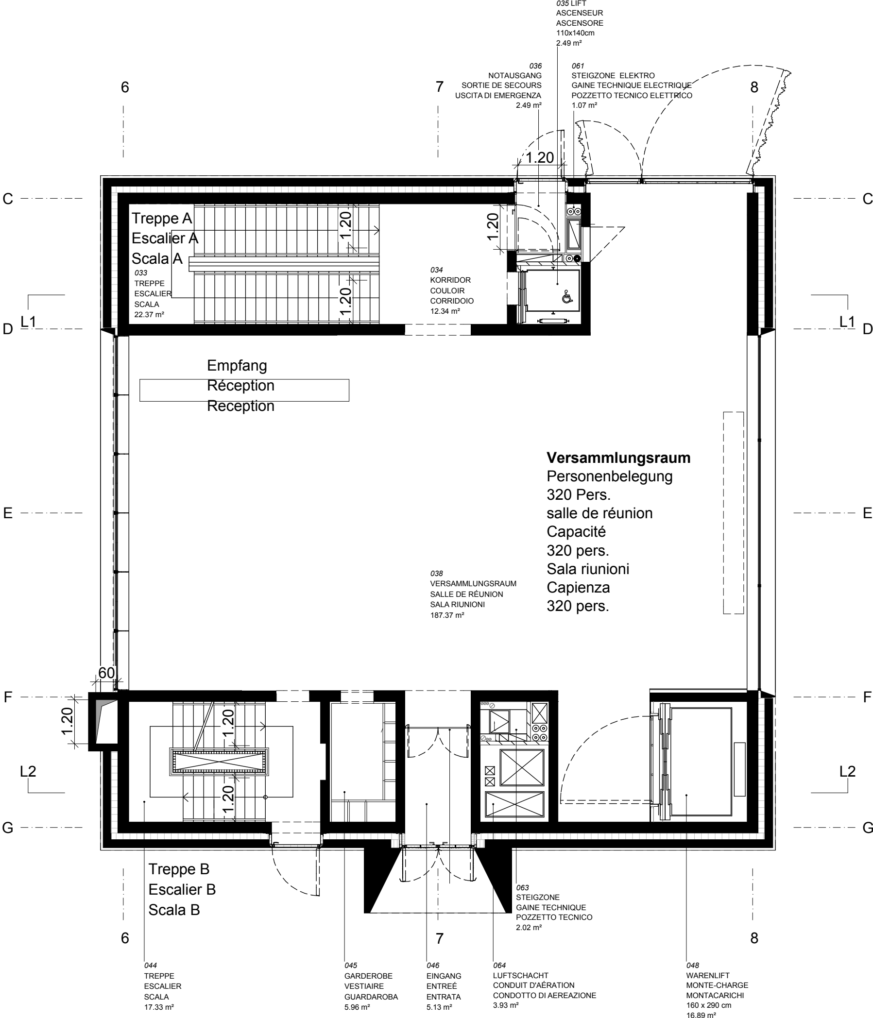
Erdgeschoss Rez-de-chaussée Pianterreno
